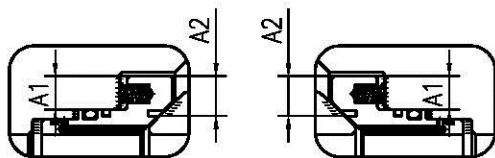
注意A2>A1 (DBB结构)
